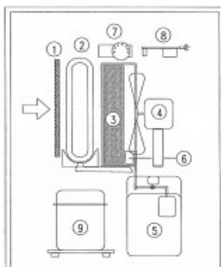
Urządzenie posiadające zbiornik pływakowy
